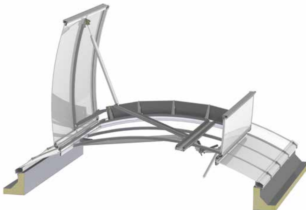
SISTEMA CI - EXUTORIO B DE LAMILUX COMO COMPUERTA DOBLE ASIMÉTRICA
